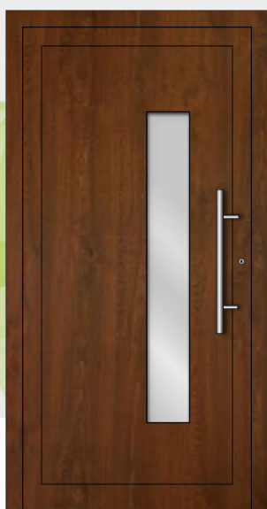
● Model: KT 3120 Typ: HPL Kolor: 2178007-167 Nussbaum Szkło: Decormat
